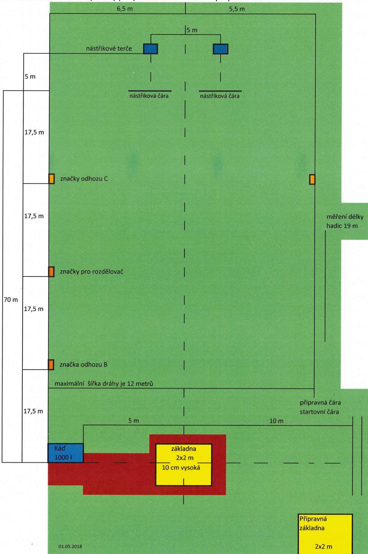
Obrázek č.1 Rozměry dráhy pro požární útok seriálu Superpohár
